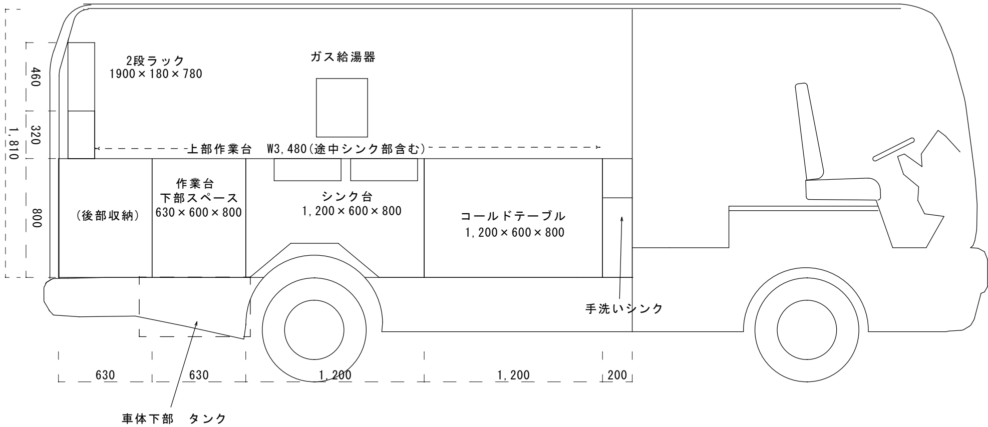
右 (運転席側)
