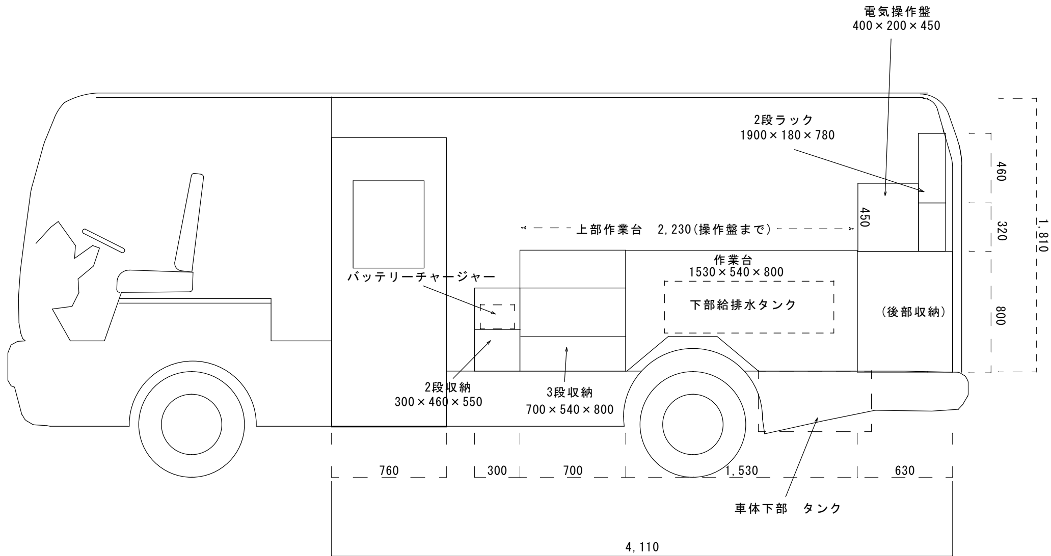
左(助手席側)
